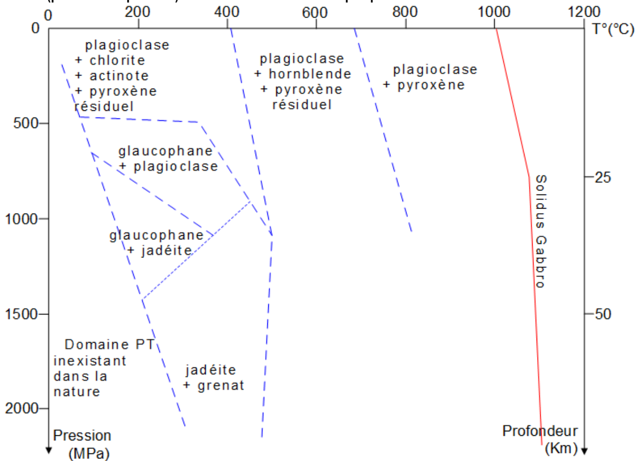
Diagramme PT (pression température) et domaines de stabilité de quelques associations minérales
